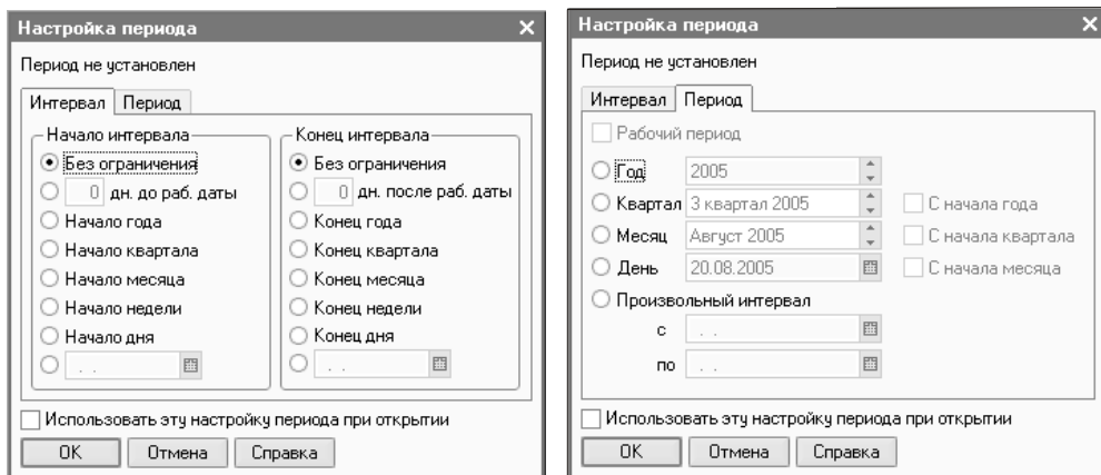
Рис. 1.16. Экранная форма настройки режима определения интервала просмотра (интервала дат) в 1С:Бухгалтерии предприятия 8.0
