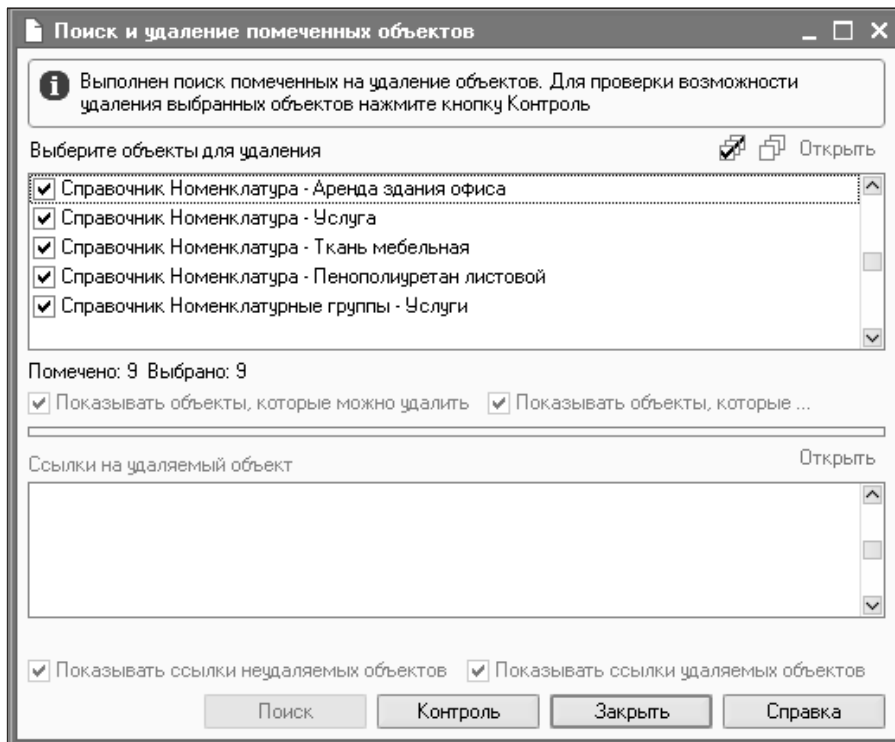
Рис. 11.4. Экранная форма режима поиска и удаления помеченных объектов в 1С:Бухгалтерии предприятия 8.0
