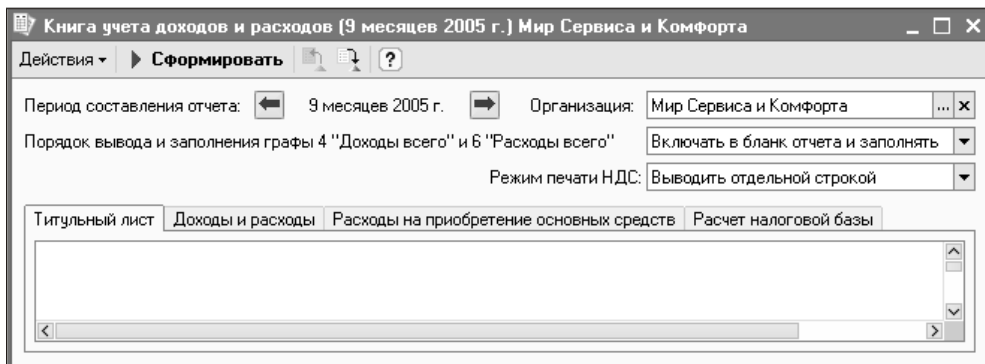
Рис. 10.2. Экранная форма настройки отчета Книга учета доходов и расходов в 1С:Бухгалтерии предприятия 8.0
