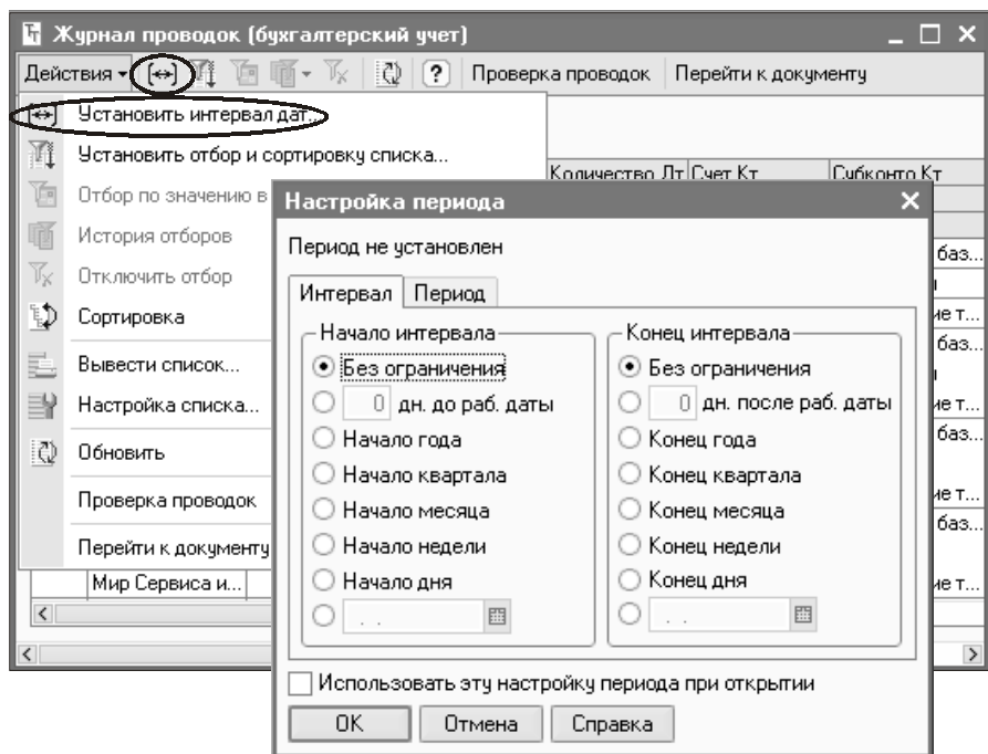
Рис. 1.14. Экранная формы закладки Журналы режима настройки параметров в 1С:Бухгалтерии — а; вызов экранной формы установки интервала в журнале 1С:Бухгалтерии предприятия 8.0 — б
