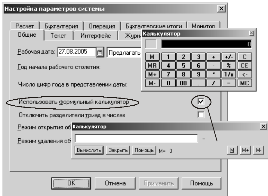
Рис. 13.1. Фрагмент экранной формы закладки Общие режима Параметры пункта меню Сервис в 1С:Бухгалтерии 7.7 с формами калькулятора и формульного калькулятора
