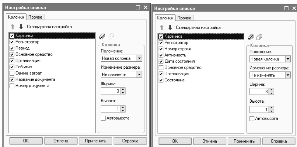
Рис. 3.9. Настройка списков регистров сведений о Событиях ОС и Состоянии ОС в рис. 3.7. и 3.8
