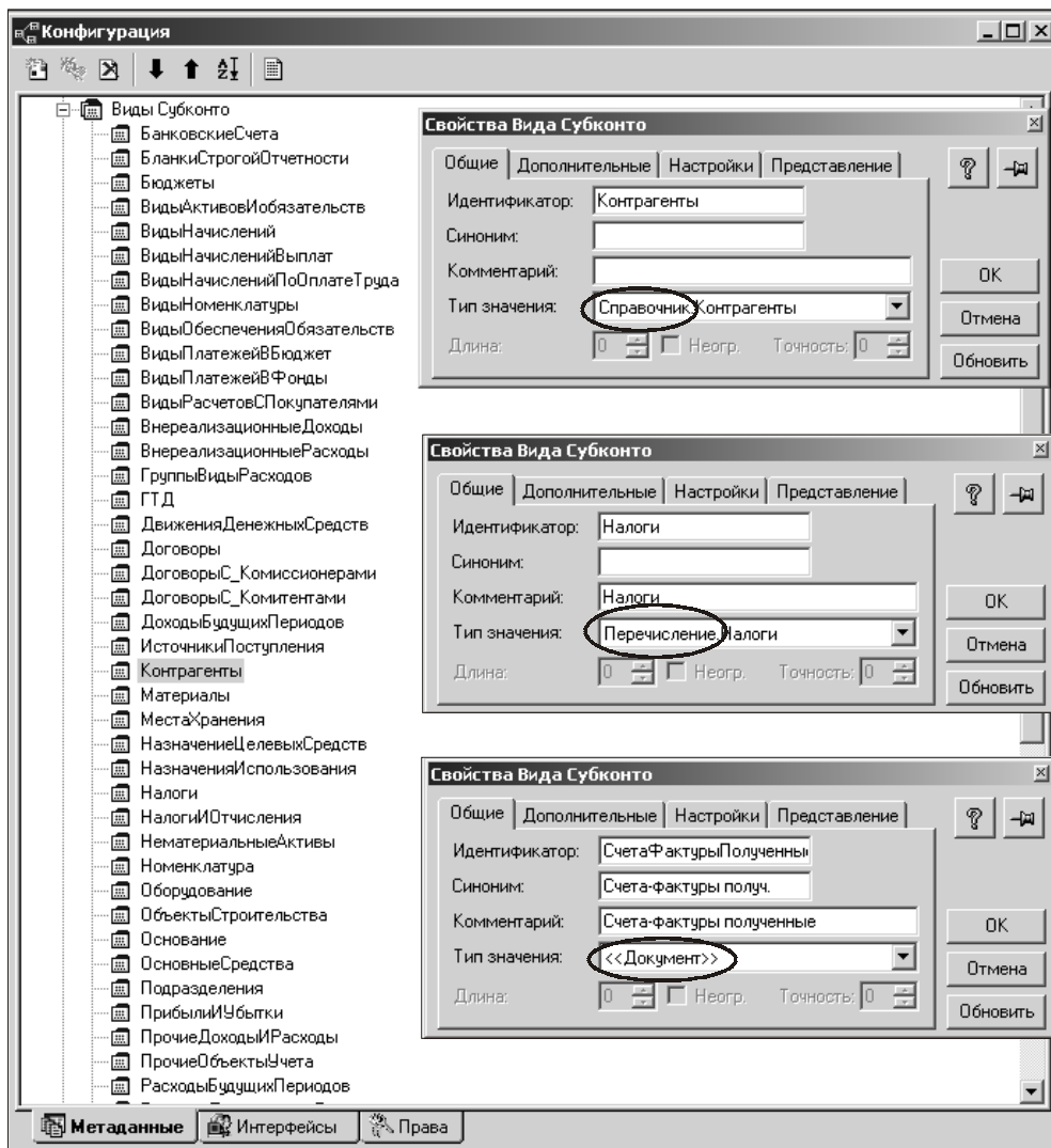
Рис. 3.52. Экранные формы настройки аналитических объектов (видов субконто) в Конфигураторе 1С:Бухгалтерии 7.7
