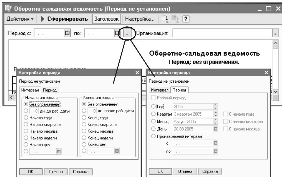
Рис. 1.17. Экранная форма закладки Бухгалтерские итоги режима настройки параметров в 1С:Бухгалтерии 7.7 — а; экранные формы режима определения периода вывода итогов в отчете 1С:Бухгалтерии предприятия 8.0 — б
